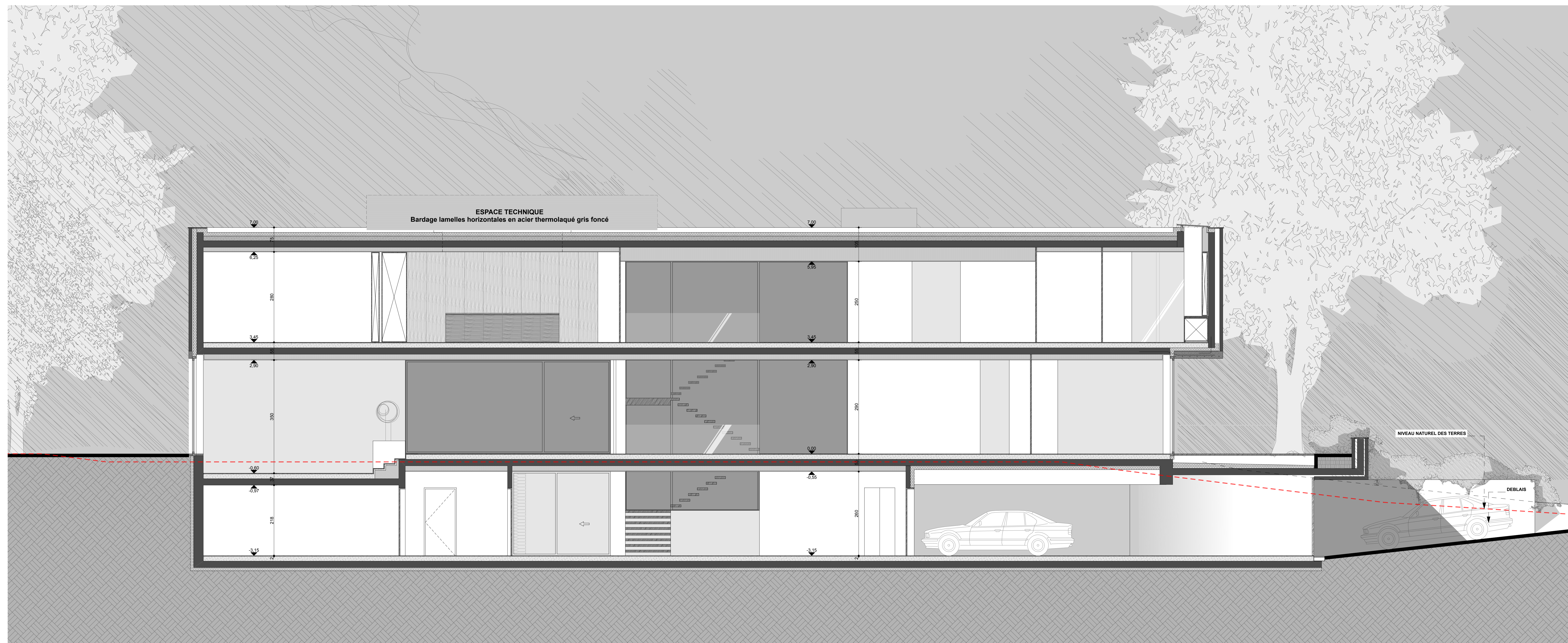
COUPE BB
