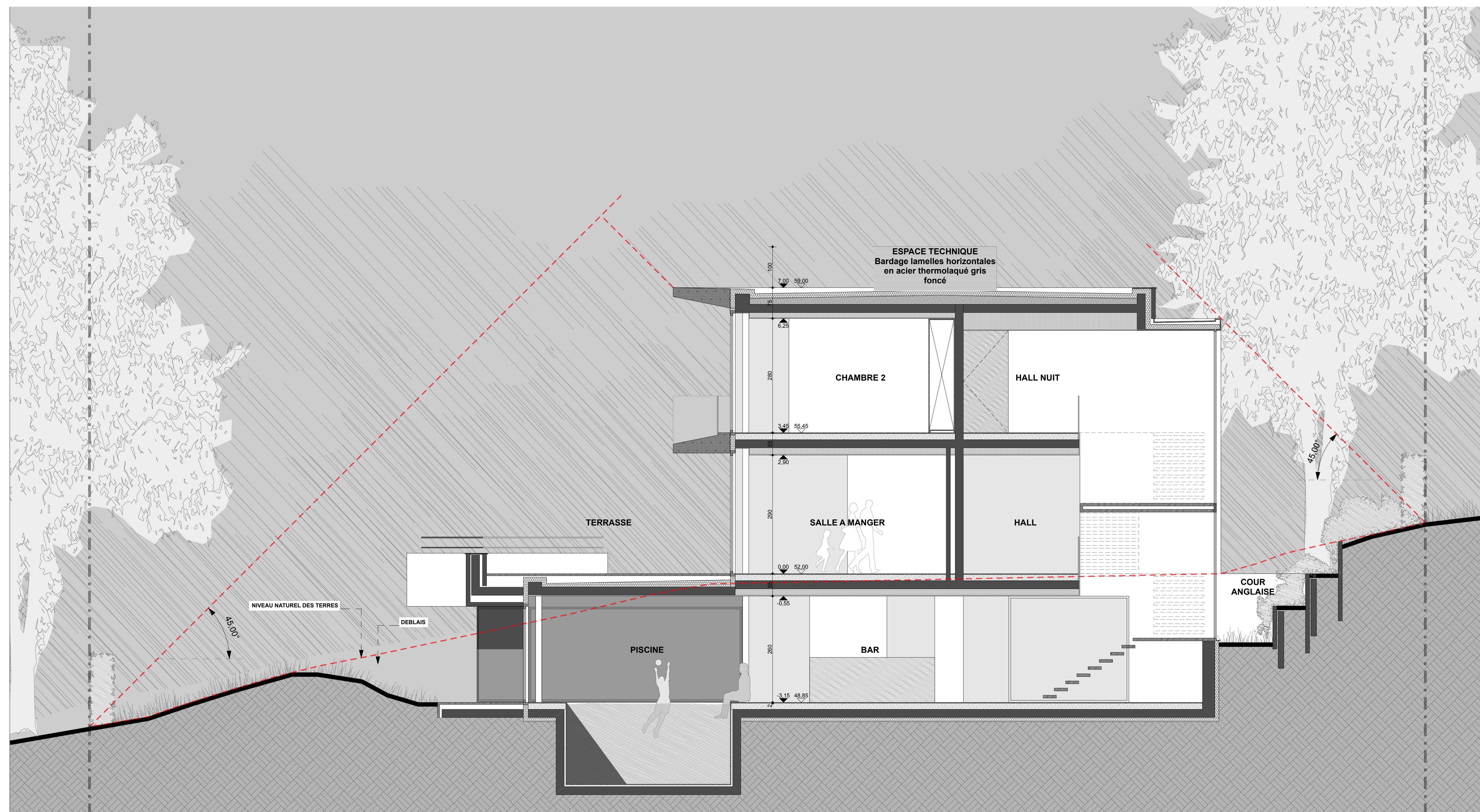
COUPE AA
